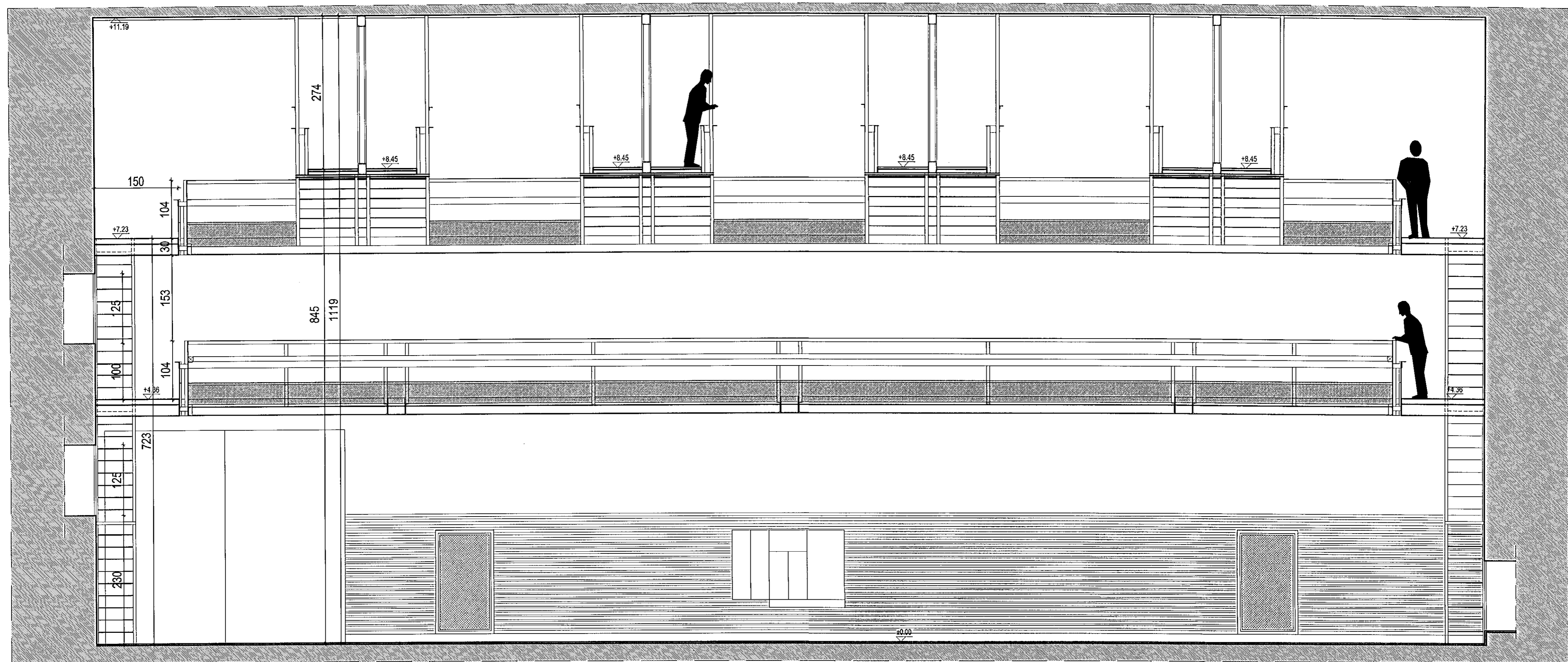
WFF WROCLAW - MAŁA HALA PRZEKRÓJ A-A SKALA 1:50
