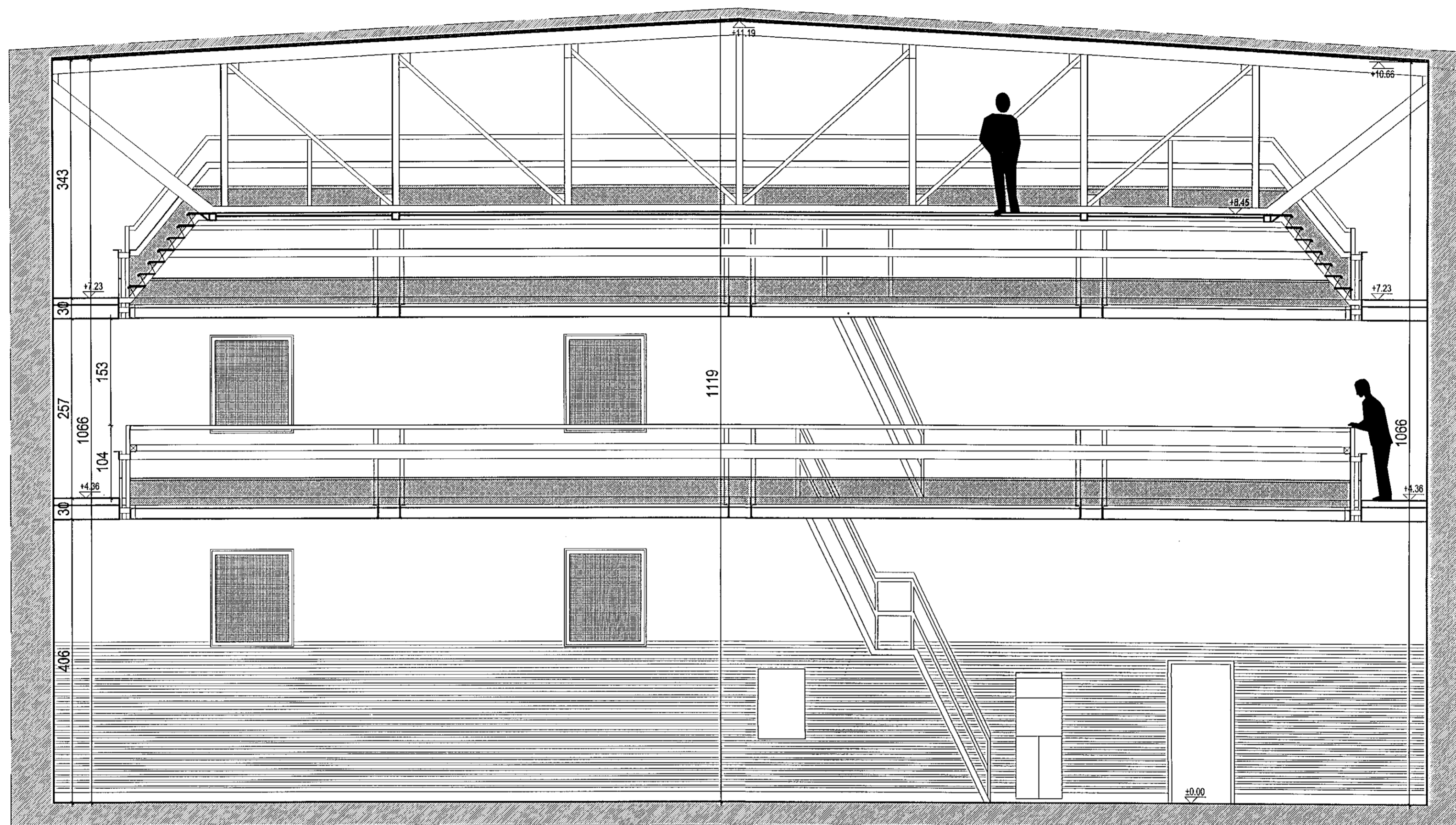
WFF WROCLAW - MAŁA HALA PRZEKRÓJ B-B SKALA 1:50
